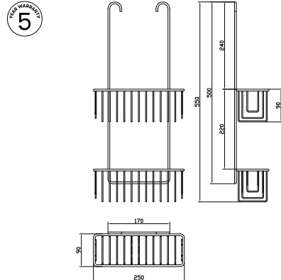
Art.nr. 30076, 30077, 30078 Blandebatterikurv Azalea Twin
