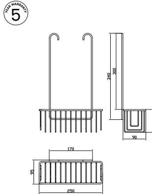
Art.nr. 30073, 30074, 30075 Blandebatterikurv Azalea Single
