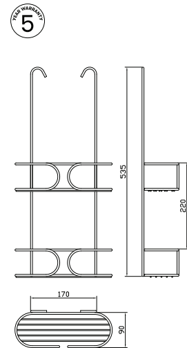
Art.nr. 30081 Blandebatterikurv Ambrosia Twin
