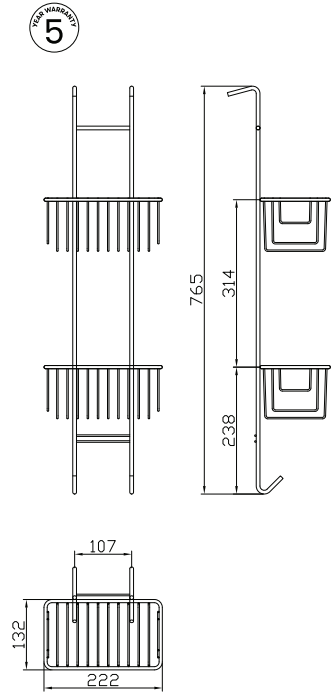
Art.nr. 30070 Dusjkurv Anemone Mini
