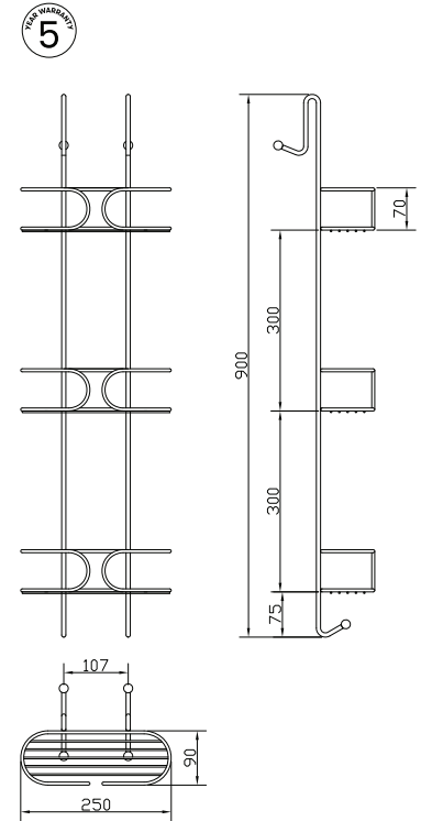
Art.nr. 30082 Dusjkurv Ambrosia Triplet
