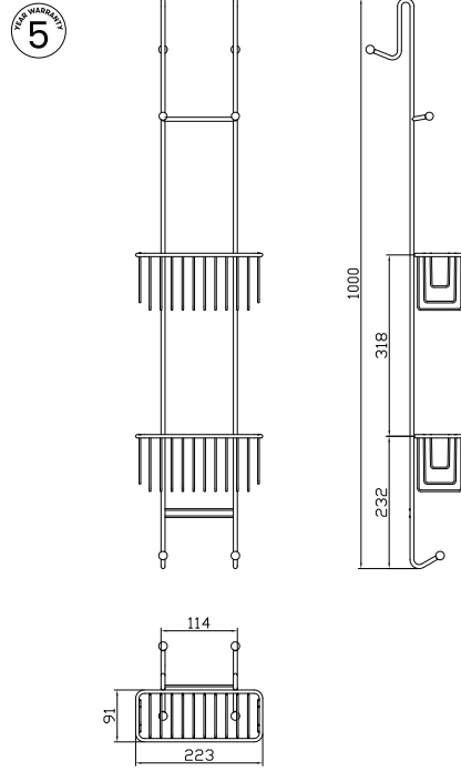
Art.nr. 30071, 30072 Dusjkurv Anemone Maxi
