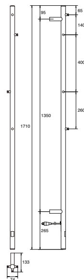
Art.nr. 30207, 30208 Håndkletørker Fern 12
